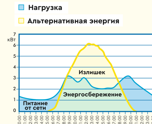
График энергопотребления типовой фермы с потреблением электроэнергии 20'000 кВт·ч/год и солнечной электростанцией на 7 кВт
